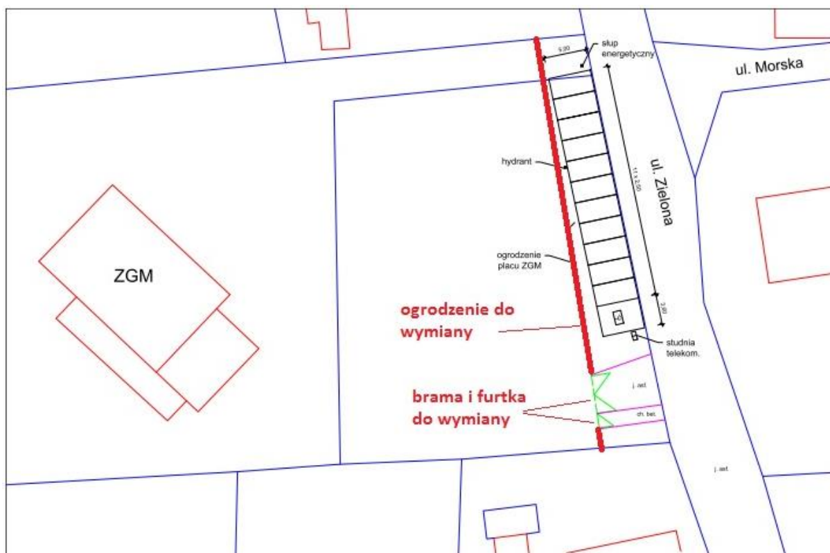
Rys. 4 – plan sytuacyjny
